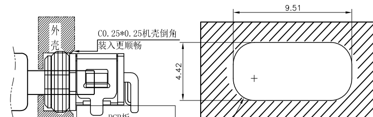
组装示意图
