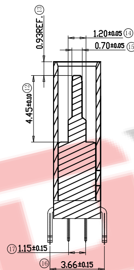
剖视图
