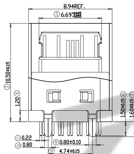
剖视图
