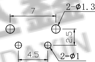
PCB. 焊接图
