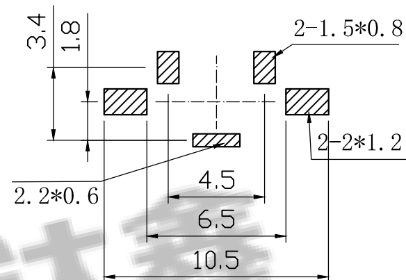
PCB. 焊接图
