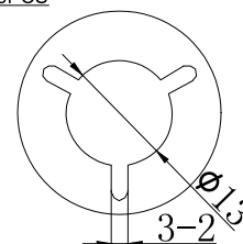
DETAIL: A 10:1
