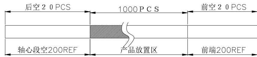
包装示意图:
