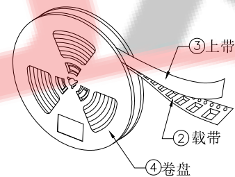
卷盘示意图
