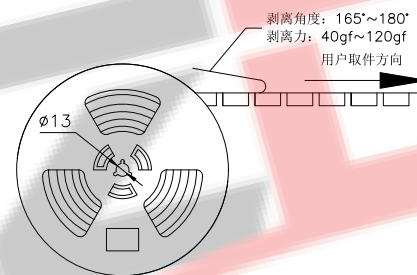
卷盘示意图
