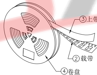
卷盘示意图
